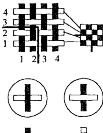
Fig. 2. Reprezentarea grafică a legăturii. Elementele țesăturii
