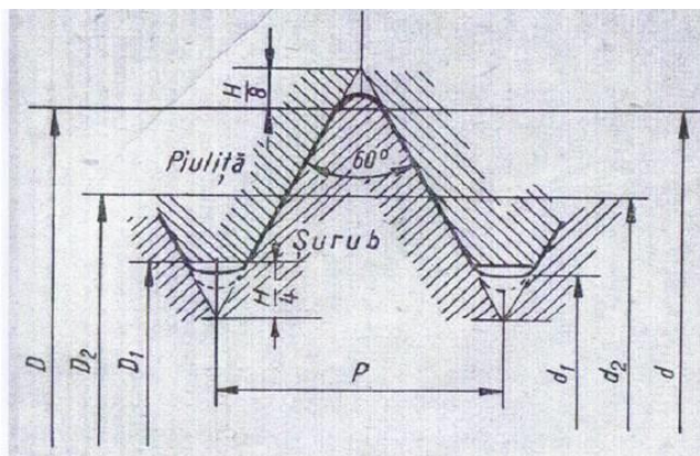
FIG. 2. FILET METRIC
