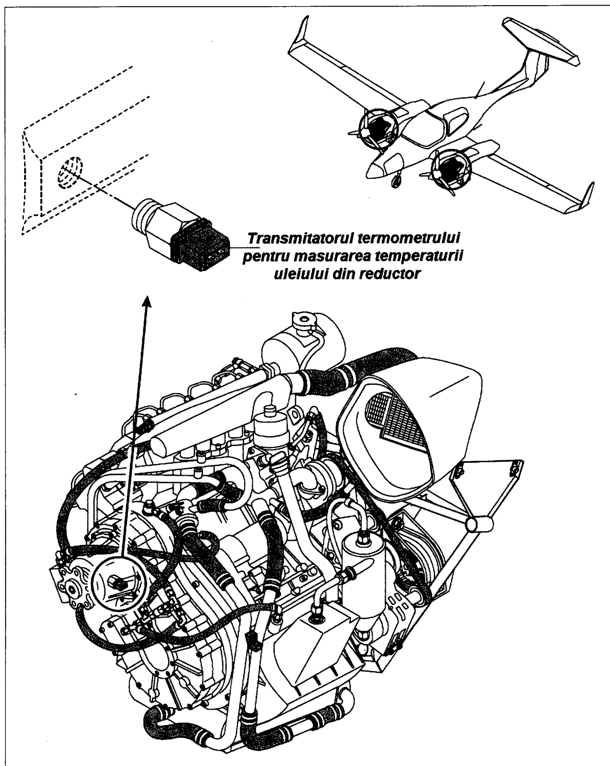
Fig. 2. Montarea transmițătorului termometrului pentru măsurarea temperaturii uleiului din reductor
