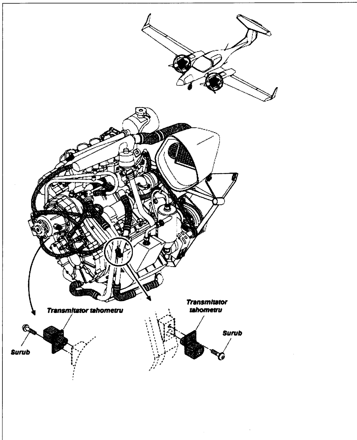
Fig. 1. Montarea transmițătorului tahometrului
