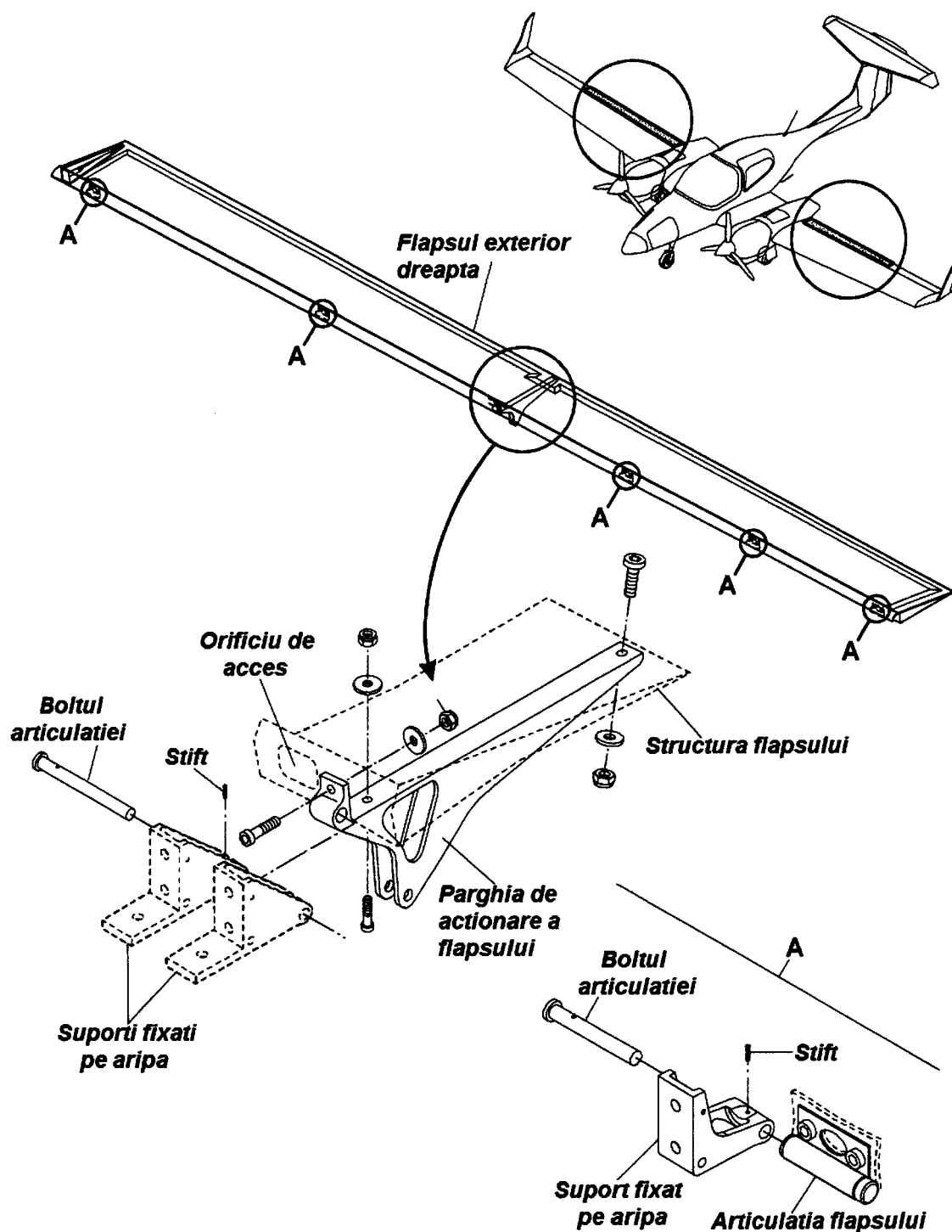
Figura 1: Montarea flapsului exterior
