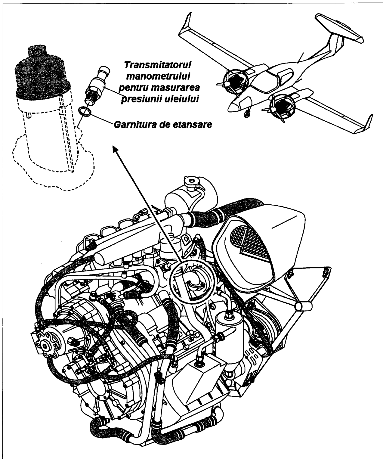
Fig. 5. Montarea transmițătorului termometrului pentru măsurarea presiunii uleiului din motor
