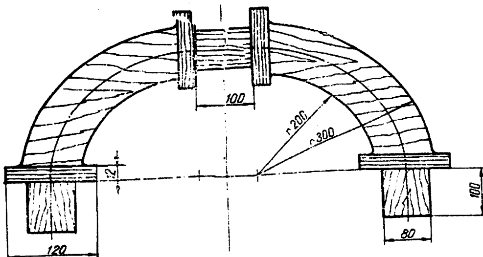
Fig.2 Executarea modelului pentru un cot de țevă
