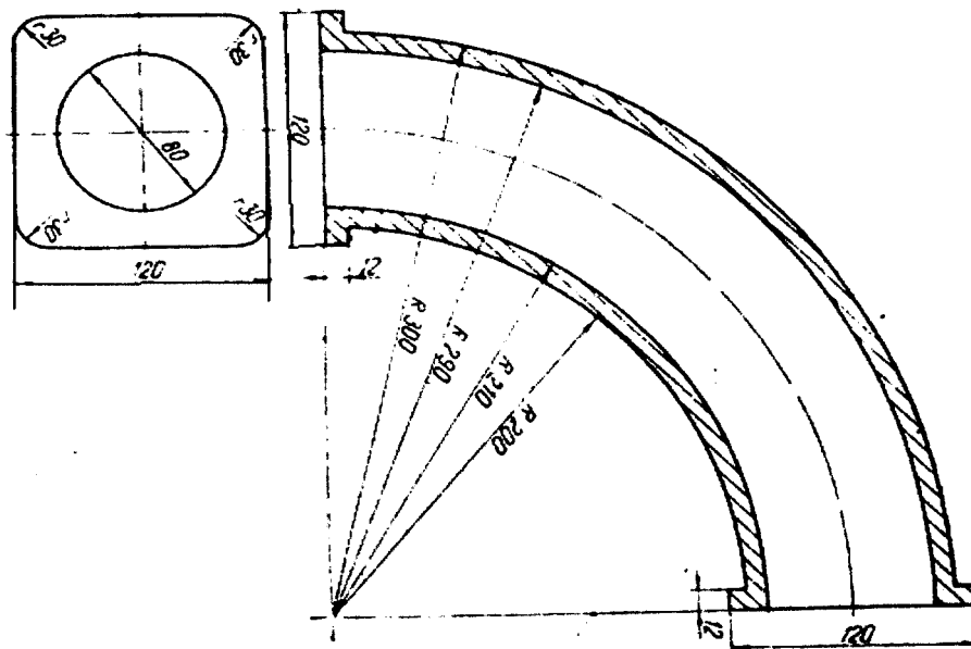
Fig.1 Cot de țevă
